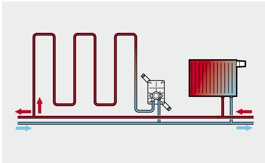
Montagebeispiel Kombibox RTL bei kombinierter Radiator-Wandheizung
